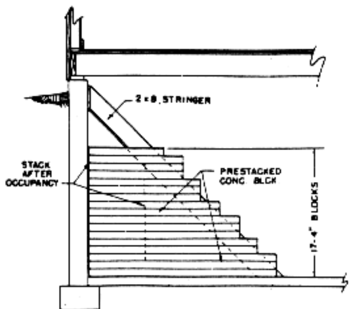
End Elevation
