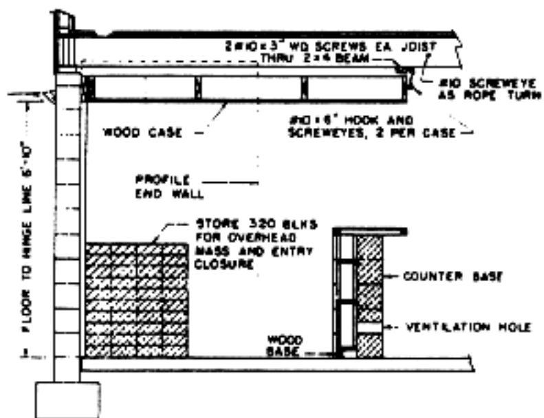
Bar Section A-1
