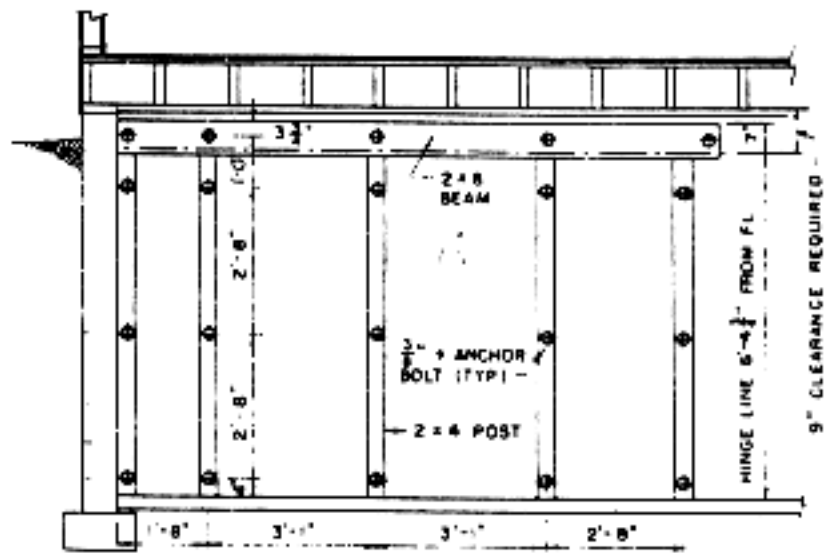
Section A-2
