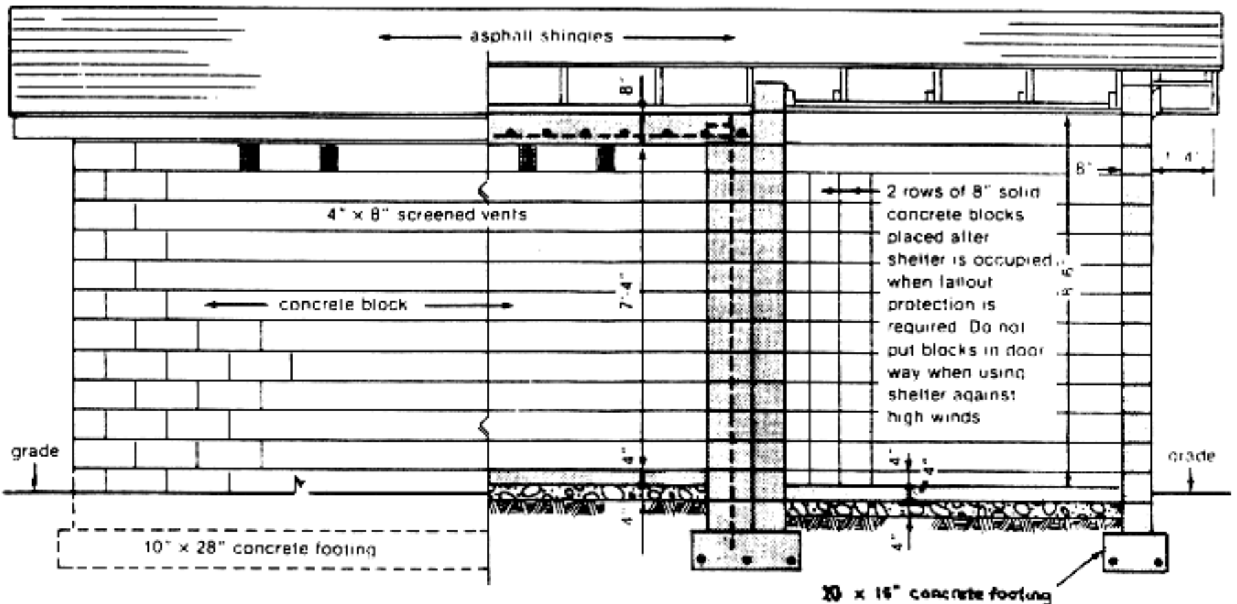
ELEVATION
