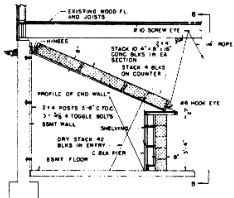
Section A-2
